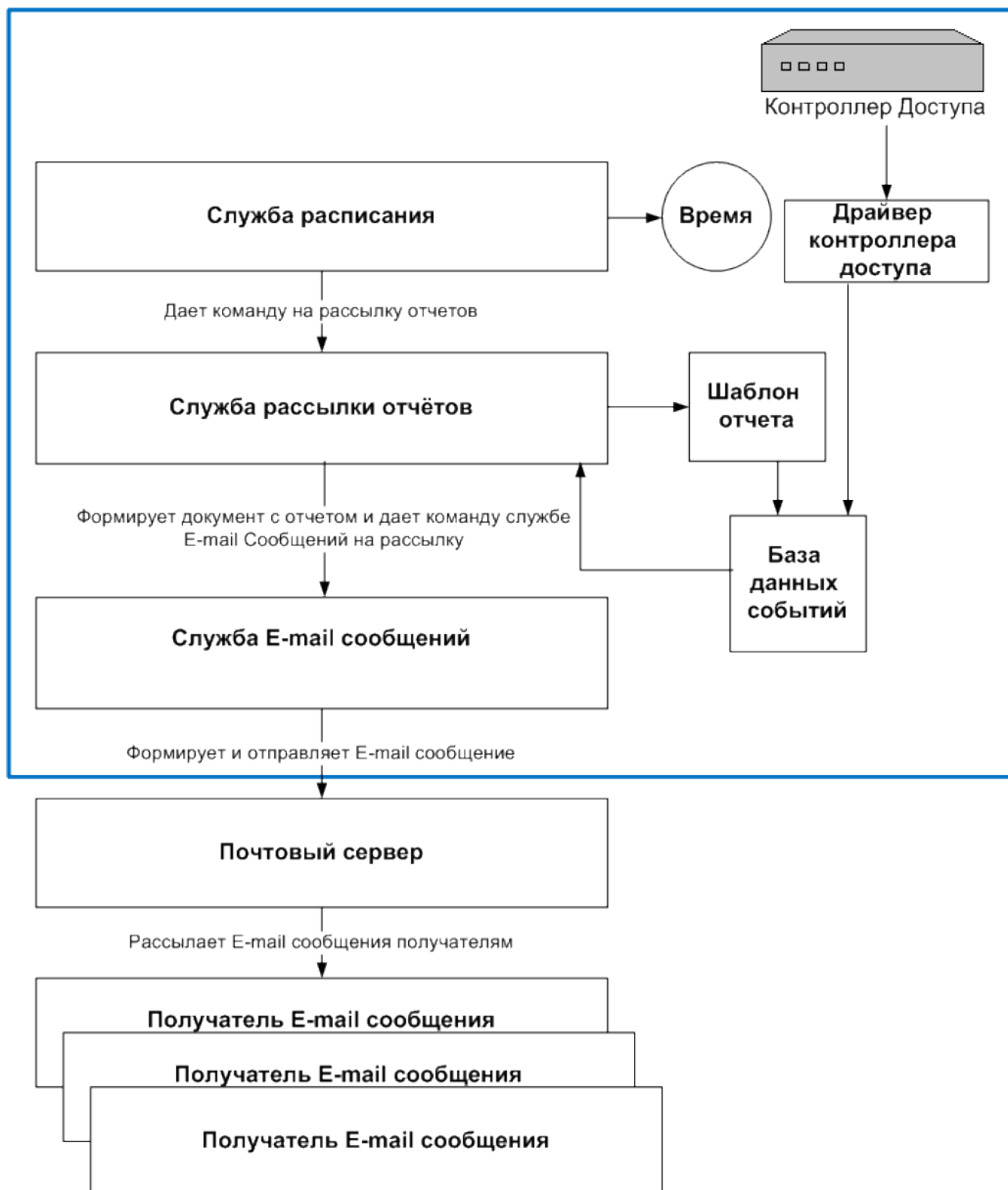
Рисунок 22 — Схема конфигурирования системы для автоматического отправления e-mail писем по опоздавшим владельцам пропусков
