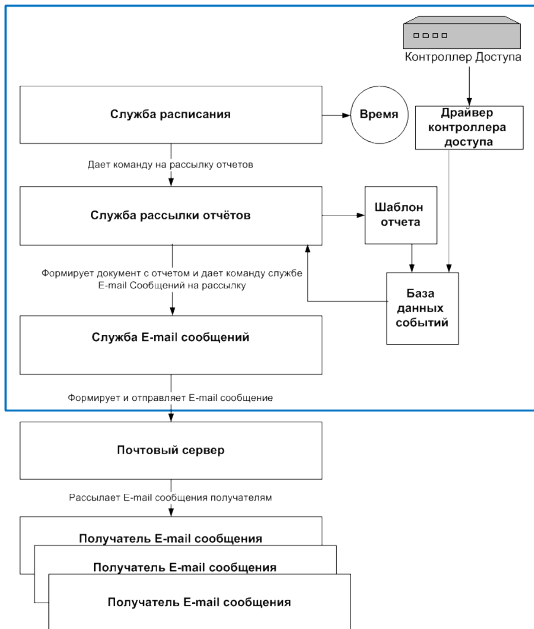
Рисунок 1 — Схема функционирования системы
